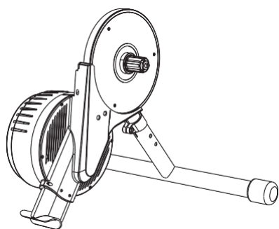
前底管安裝完成示意图
